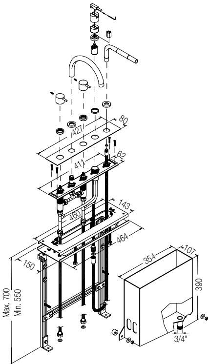
Combinaison complète système extractible avec boîte de sécurité (type BK).
